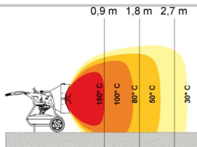
Funktionsprincip
