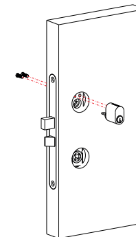
Paso 2. Ensamble el cilindro.
