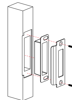
Stap 3. Boor een gat voor de sluitplaat/sluitkast
