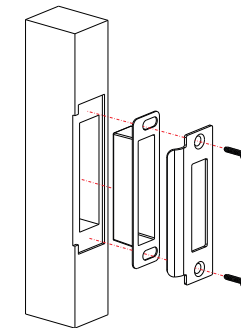
Paso 3. Taladre el orificio para la placa/caja de cierre.
