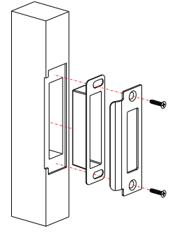
Étape 3. Percez un trou pour la gâche/boîte
