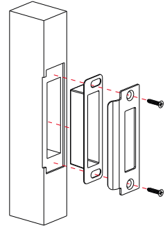
Schritt 3. Bohren Sie ein Loch für die Schließplatte/den Schließkasten.
