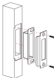
Étape 3. Percez un trou pour la gâche/boîte
