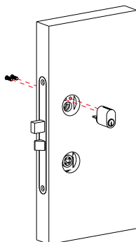
Trin 2. monter medbringer og cylinderen
