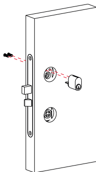
Étape 2. Assemblez le cylindre
