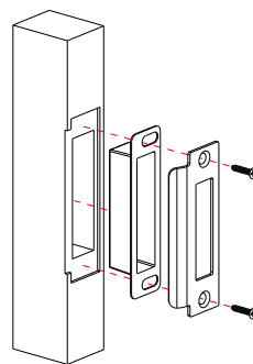
Paso 3. Taladre el orificio para la placa/ caja de cierre.
