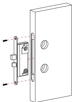
Étape 1. Assemblez la mortaise
