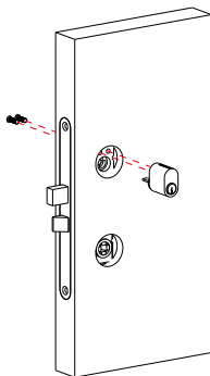
Paso 2. Ensamble el cilindro.
