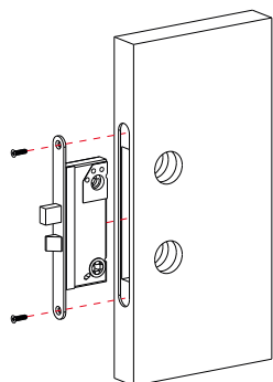
Trin 1. isæt låsekassen
