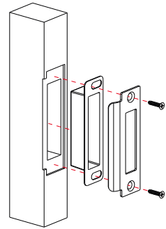
Stap 3. Boor een gat voor de sluitplaat/ sluitkast
