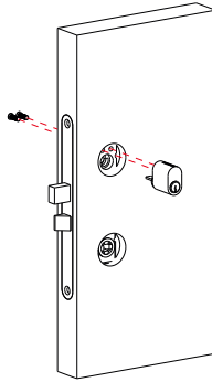
Schritt 2. Montieren Sie den Zylinder.
