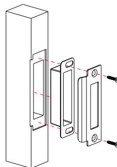
Trin 3. monter slutblik i dørkarm
