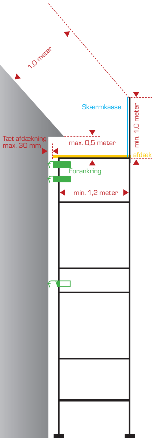
Fig. 1 Dobbelt forankring med muranker på murbukkens overligger. Monter forankring inden platforme.
