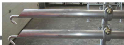
Fig. 2 Dobbelt forankring med rørfastgørelse på overliggerens lodrette søjle. Brug en rørfastgørelse samt en dobbelt fast kobling 48/34 mm (varenr: 18SFF105-3448)
