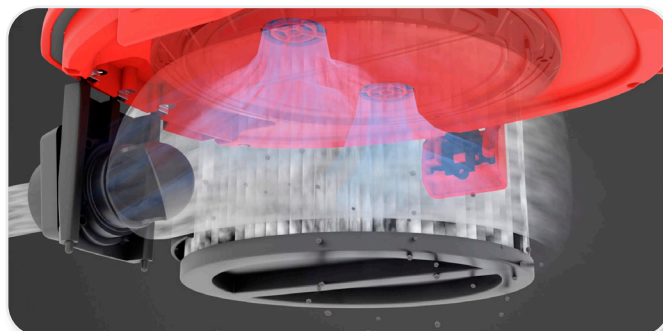
Den består af to uafhængige filterkamre, der bliver renset på skift. Luftstrøm og sugekraft forbliver således på et konstant højt niveau, selv under rensning, hvilket garanterer permanent sug.
